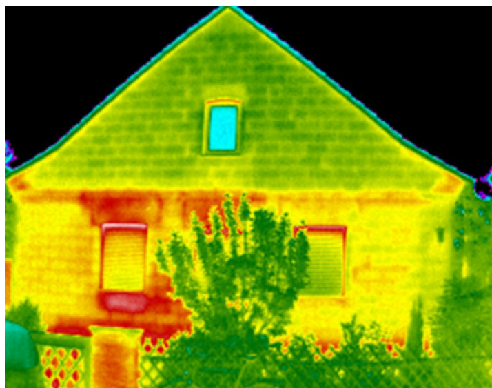
Im Wärmebild lässt sich erkennen, dass über Rollladenkästen und Fensterbänke der linken Haushälfte viel Wärme nach draußen gelangt (im Bild rot gefärbt). (Foto: Verbraucherzentrale Rheinland-Pfalz e.V.)
